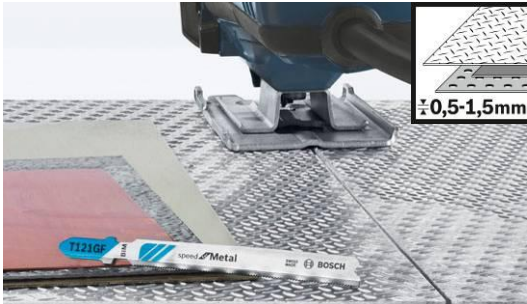
T121GF za izuzetno tanke limove.
